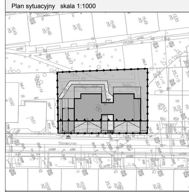
Plan sytuacyjny skala 1:1000
